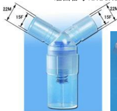
型番:Ku-004(54111000) ウォータートラップ(自動シール弁式)
